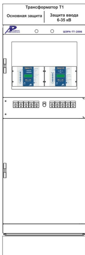
Шкаф защит трехобмоточного трансформатора и АУВ стороны НН ШЭРА-ТТ-2006 (БПВА.656457.459, БПВА.650645.001 ТУ)
